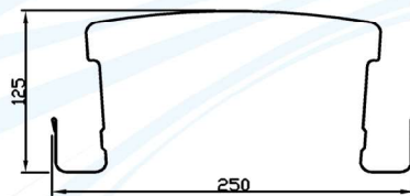
几字形栽培槽 Gutter for tomato (常用于种植番茄等作物)
